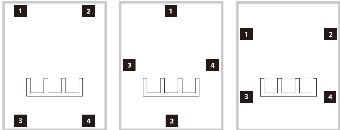
使用四个S10D的推荐低音炮放置选项
