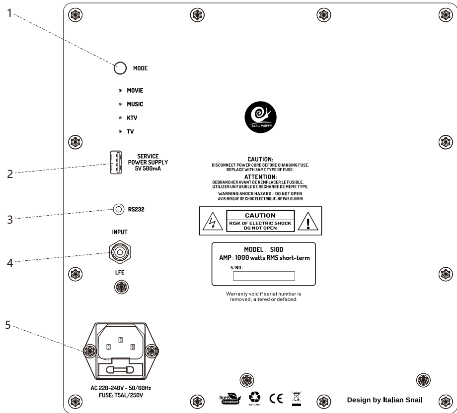
5：后面板功能说明
