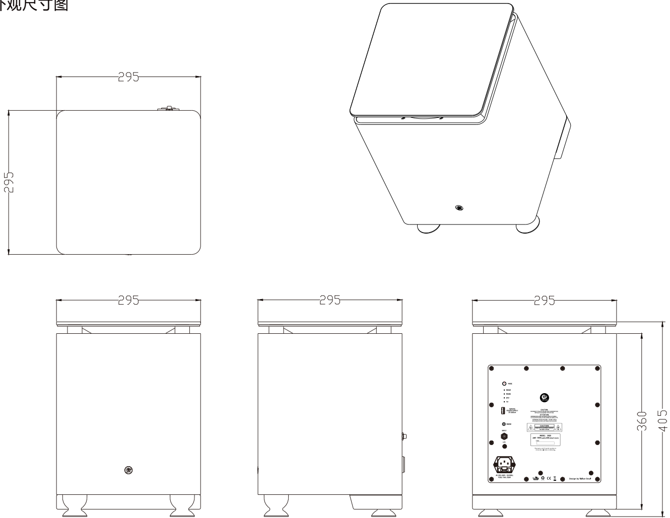
6：外观尺寸图
