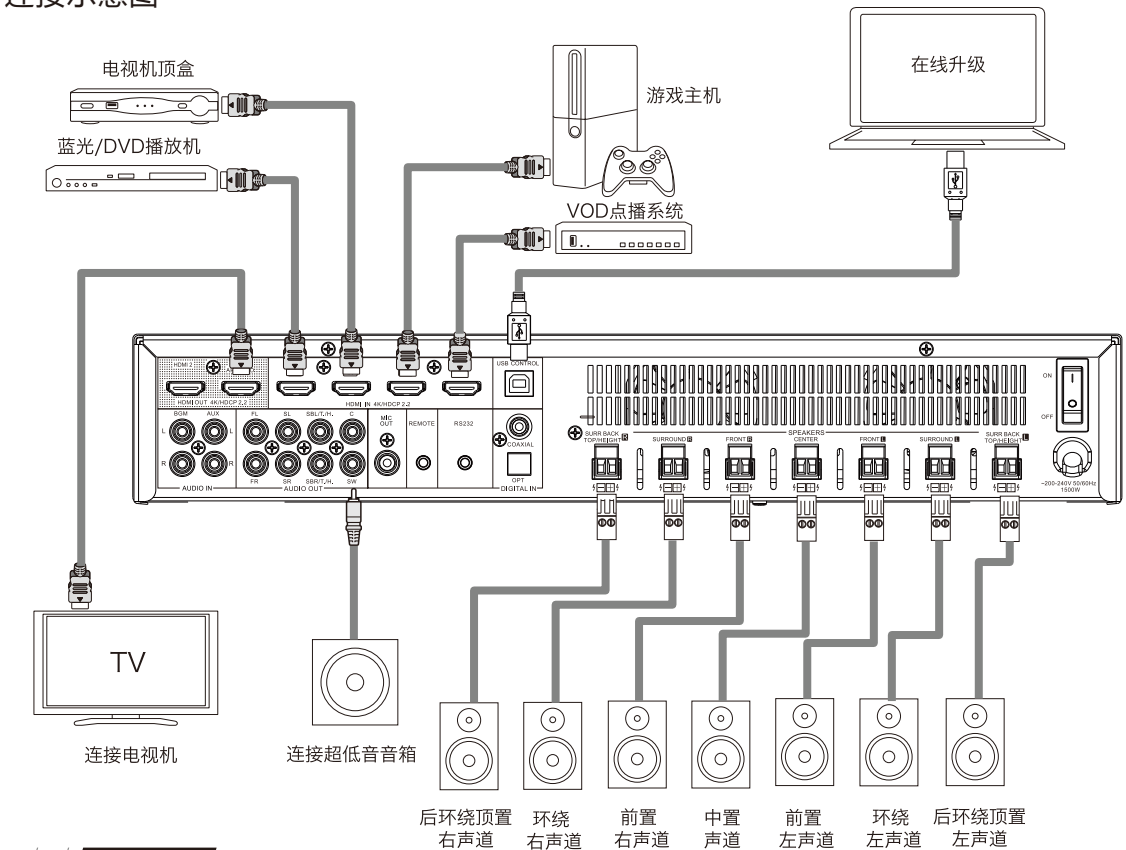
连接示意图
